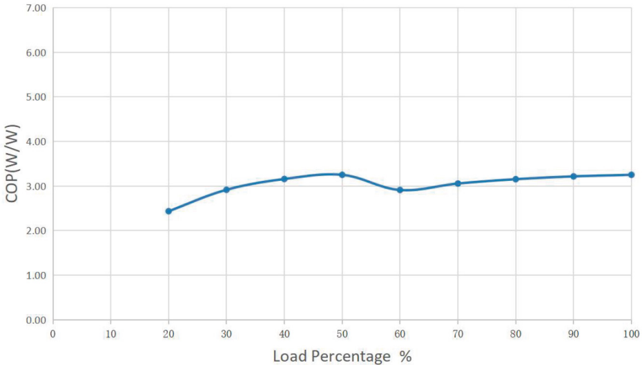
Ten Points Parameters(Constant Ambient Temp.)
